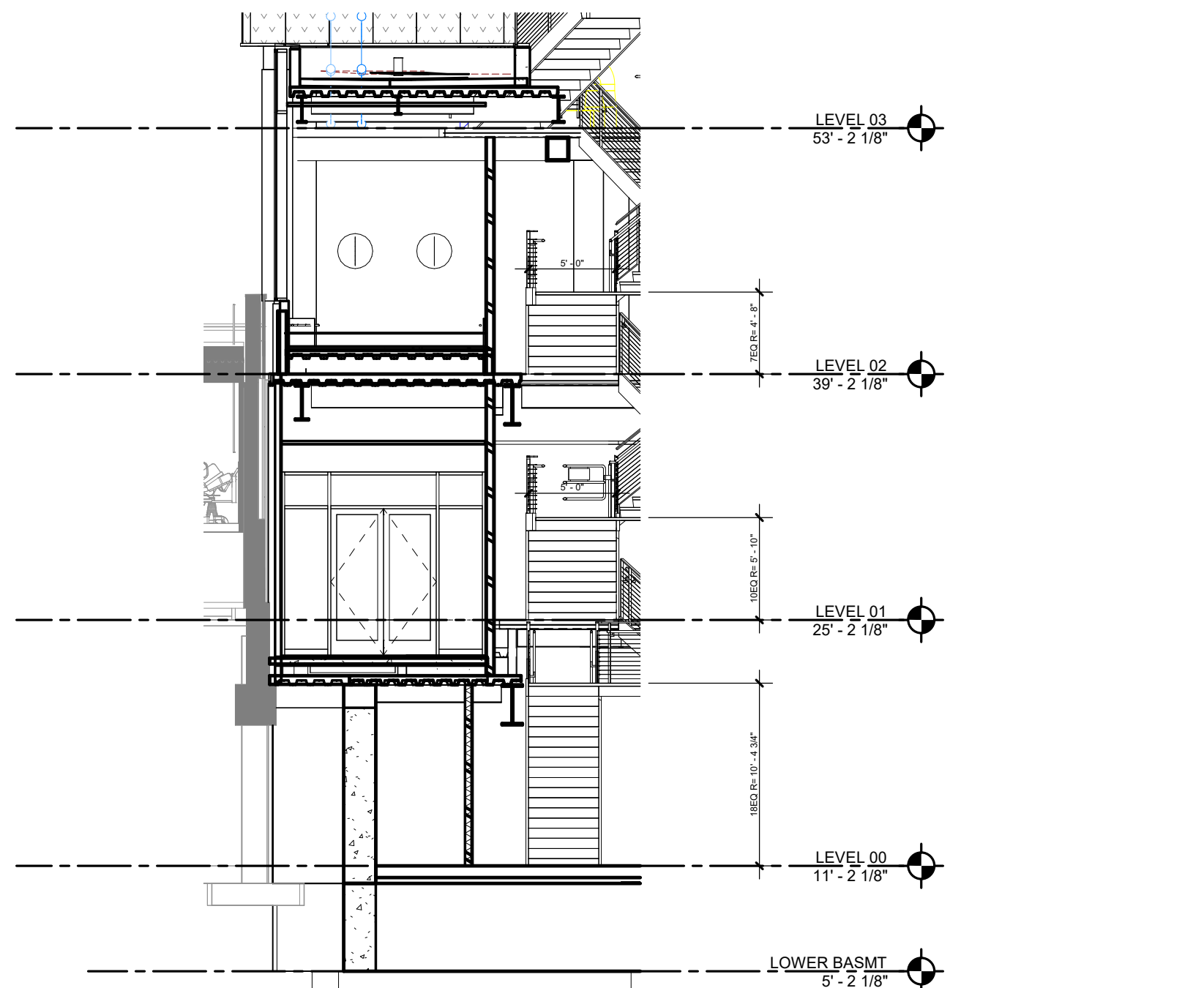
04 SE STAIR SECTION 04 1/8" = 1'-0"
