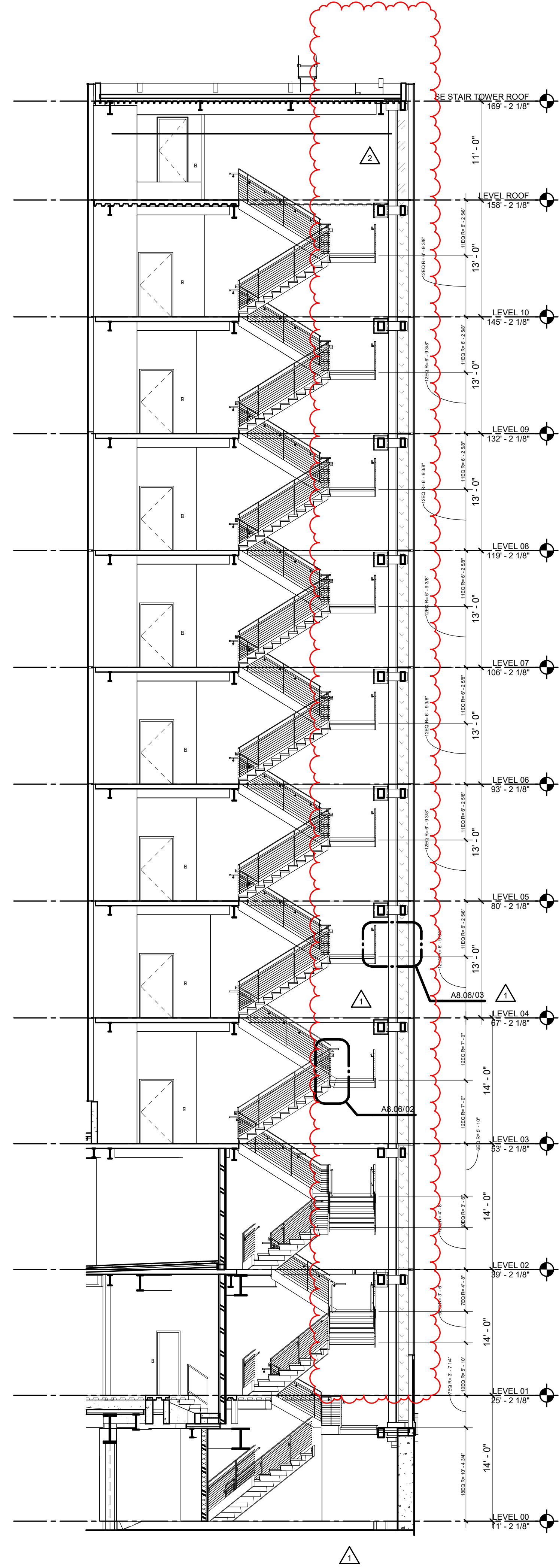
01 SE STAIR SECTION 01 1/8" = 1'-0"
