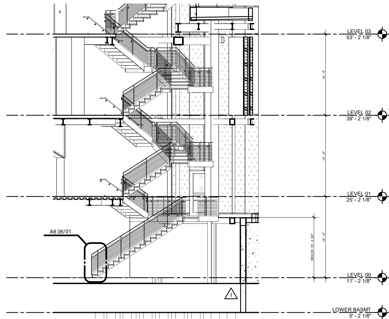
03 SE STAIR SECTION 03 1/8" = 1'-0"
